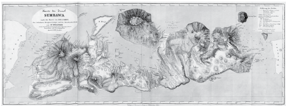
Fig. 2. Mappa di Sumbawa con il vulcano Tambora, allegata al volume di Zollinger. (Consultabile in E-lib.ch (Elektronische Bibliothek Schweiz), ETH-Bibliothek Zürich, Rar 5880, Persistenter Link: http://www.e-rara.ch/zut/content/titleinfo/3285073 ).
